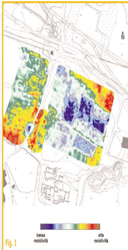
Tomografia dell'area archeologica di Cuma.
